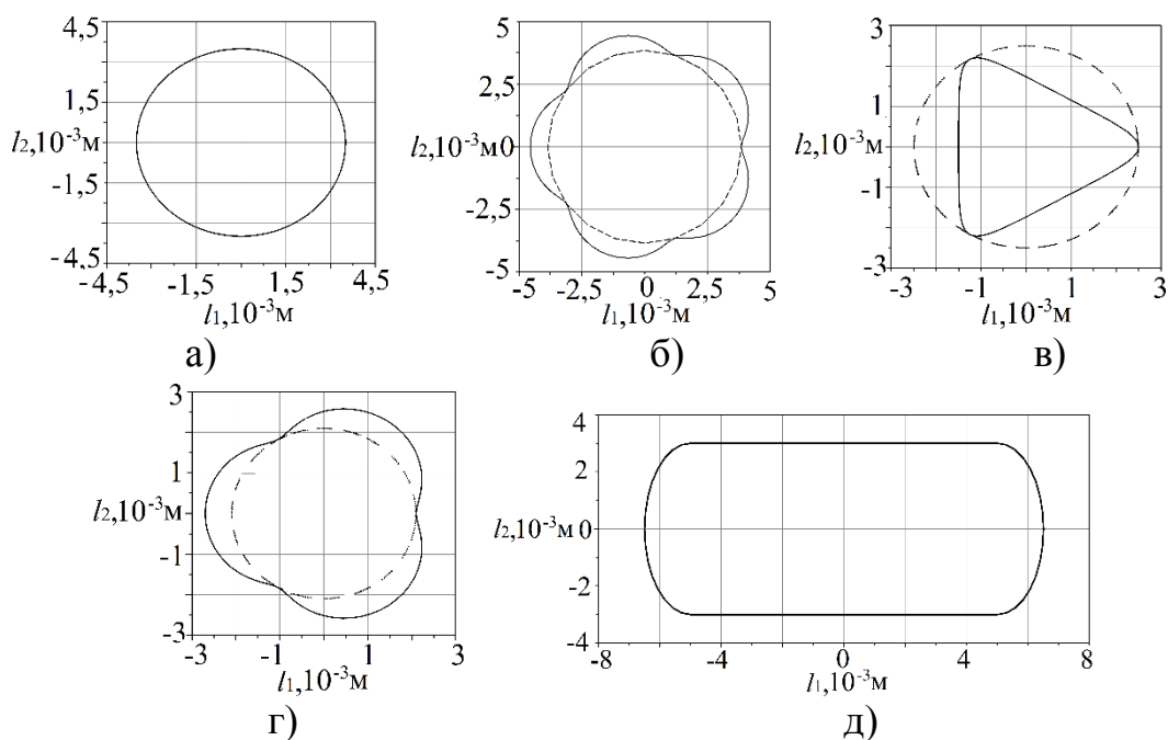
Рис. 5. Геометрія отворів віброрешіт: а – круглі ( R_0=0,0035 \text{ м} ; k=0 ); б – з п'ятипелюстковими епіциклоїдними активаторами ( R_0=0,0035 \text{ м} ; k=5 ); в – трикутні ( R_0=0,003 \text{ м} ; k=3 ); г – з трипелюстковими епіциклоїдними активаторами А ( R_0=0,0018 \text{ м} ; k=3 ); д – з прямокутними об'ємними активаторами ( R_s=0,016 \text{ м} , r_m=0,005 \text{ м} ).
