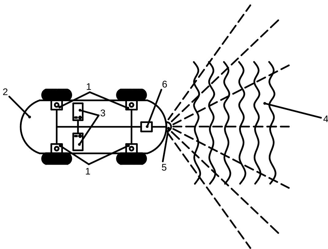
Рис. 1. Схема елементів транспортного засобу: 1 – магнітоелектричні амортизатори, 2 – транспортний засіб, 3 – акумуляторні батареї, 4 – проїзна частина, 5 – давачі, 6 – блок керування.
