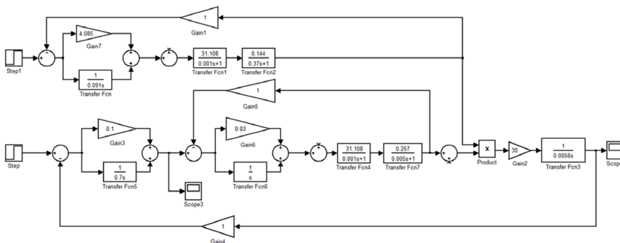
Рис. 1. Імітаційна модель системи в програмі Simulink.
