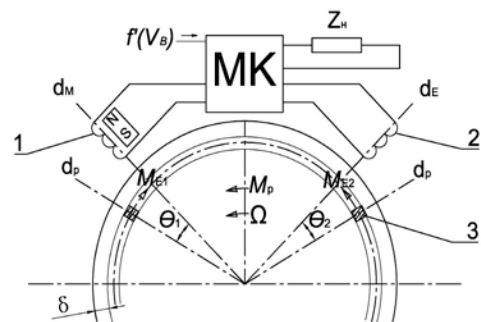
Рис. 1. Узагальнена модель бездавачевого індукторно-реактивного електромехатронного перетворювача.
