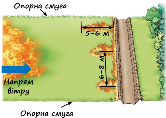
Рис.8. Відпал способом гребінки
