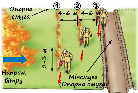
Рис. 9. Відпал способом випереджувального вогню
