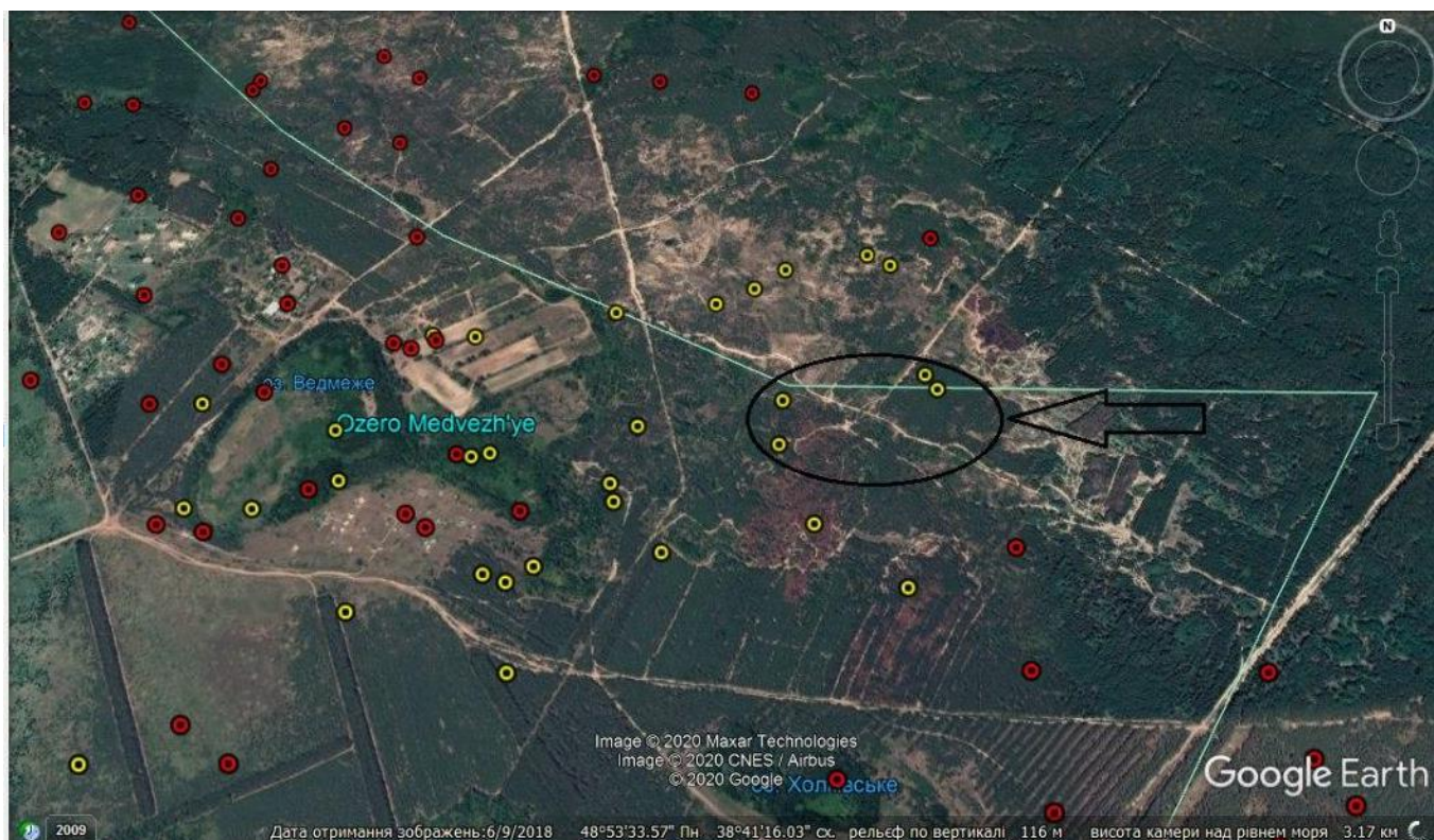
Рис. 2. Жовтим кольором позначено осередки загорання біля озера Ведмеже, червоним – пожежі протягом 7-12 липня (FIRMS та Google Earth Pro)
