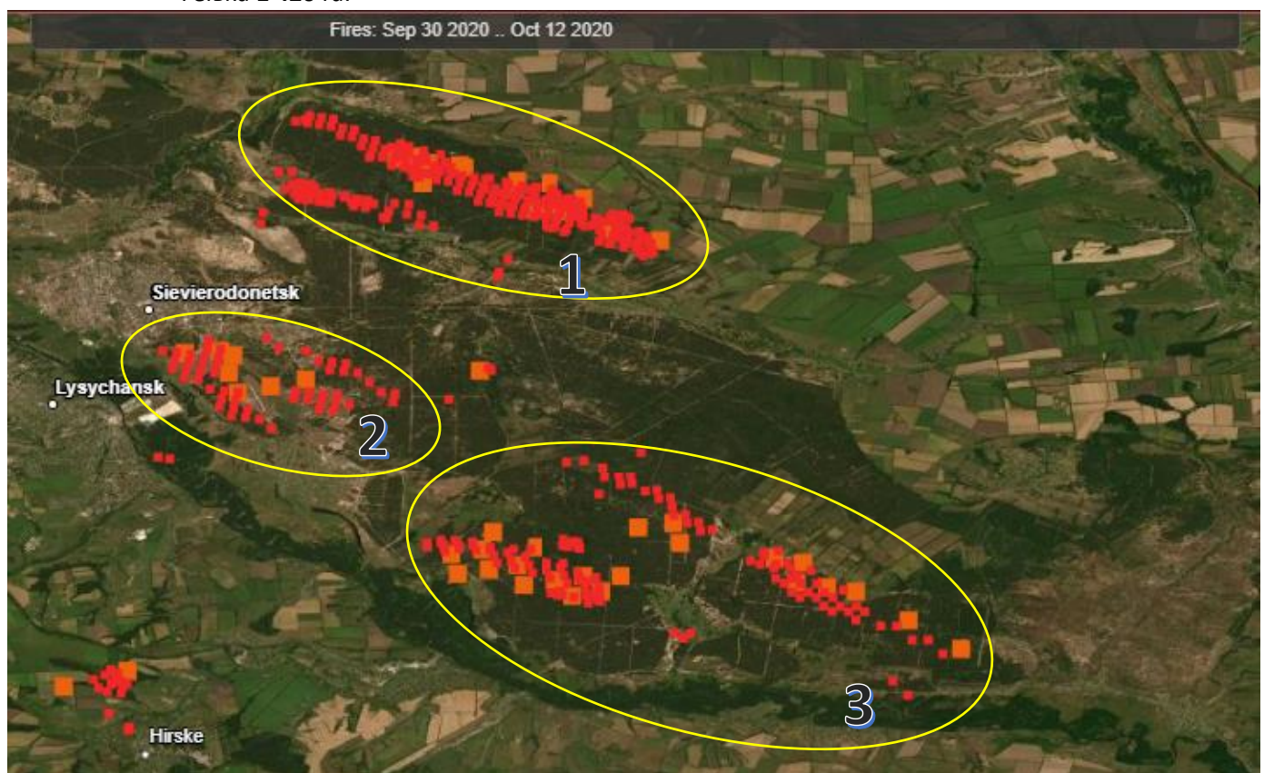
Рис. 6. Випадки пожеж біля населених пунктів Луганської області: 1 – Боровеньки, Гаврилівка, Олександрівка 4 515 га, 2 – Воронове 3 614 га, 3 – Боброве, Муратове, Капітанове, Кряківка 7 723 га (FIRMS https://firms.modaps.eosdis.nasa.gov/map/#t:adv;d:2020-09-30..2020-10-12;l:countries;@38.7,48.9,10z )
