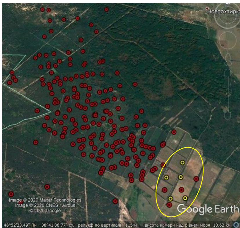
Рис. 1. Жовтим кольором позначено осередки загорання біля с. Капітанове, червоним – пожежі протягом 7-12 липня (FIRMS та Google Earth Pro)
