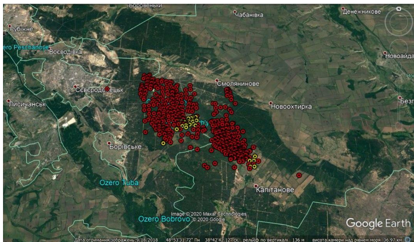
Рис. 3. Жовтим кольором позначено два осередки загорання протягом 6 липня, червоним – пожежі протягом 7-12 липня (FIRMS та Google Earth Pro)
