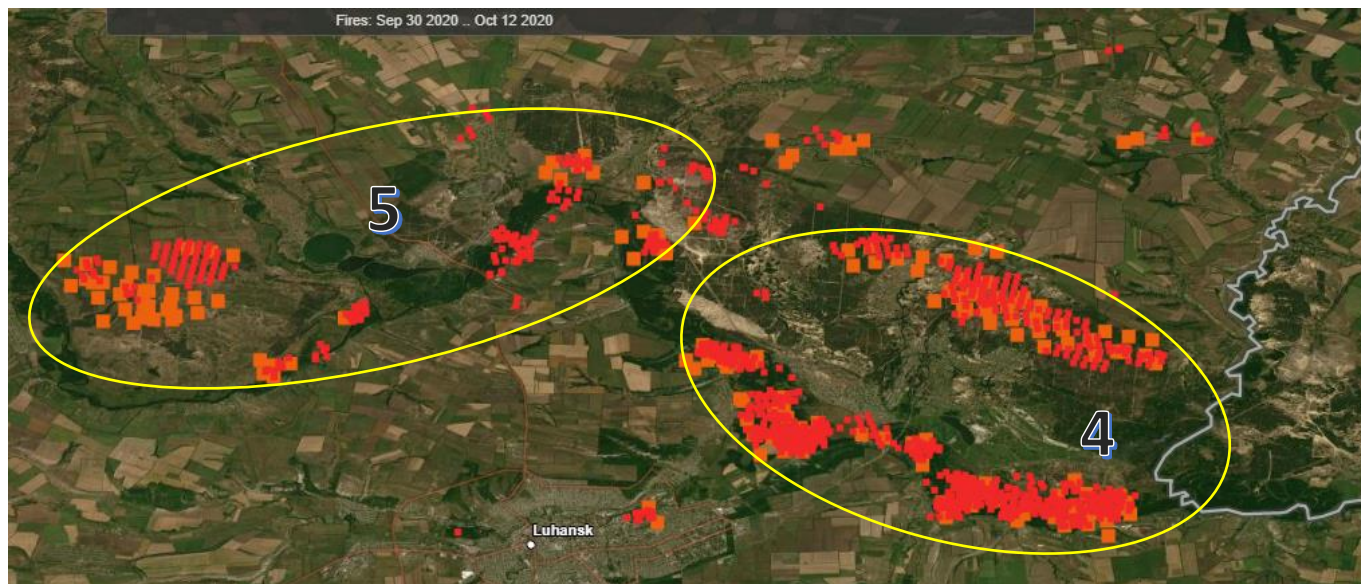
Рис. 7. Випадки пожеж біля населених пунктів Луганської області: 4 – Вільхове 10 303 га, 5 – Піщане, Нижньотепле, Артема, Геївка 1 420 га (FIRMS https://firms.modaps.eosdis.nasa.gov/map/#t:adv;d:2020-09-30..2020-10-12;l:countries;@39.3,48.7,11z )
