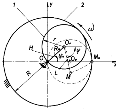
Рис. 1. Розрахункова схема визначення параметрів планетарного механізму приводу ножа різального апарату:
