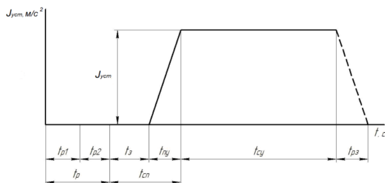
Рис. 1. Гальмівна діаграма автомобіля: t_p – тривалість реакції водія; t_{сп} – тривалість спрацьовування гальмівної системи; t_{cy} – тривалість гальмування зі сталим уповільненням; t_{p3} – тривалість розгальмування
