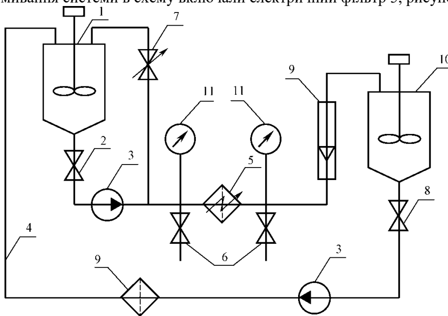
1 - витратний бак; 2, 8 - крани; 3 - насос; 4 - трубопровід; 5 - випробовуваний електричний фільтр; 6 - крани відбору проб; 7 - витратомір; 9 - технологічний фільтр; 10 - допоміжний бак; 11 - манометр.
