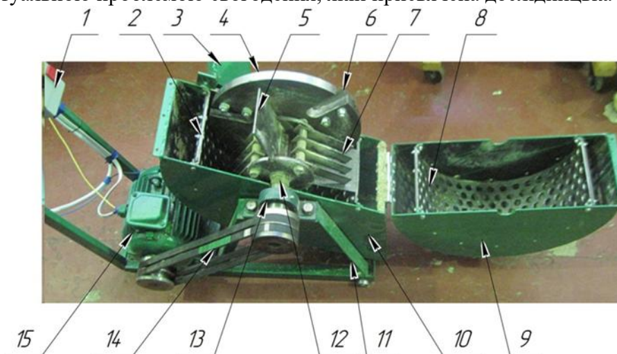
Рис. 1. Загальний вигляд малогабаритного подрібнювача деревної зелені для корму тварин: 1 – пульт керування; 2 – планка кріплення решета; 3 – завантажувальний бункер;
