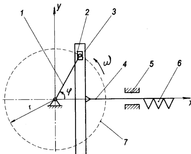
Рис. 3. Схема кінематична «синусоїдного» приводу різального апарату жаток низького зрізу:
