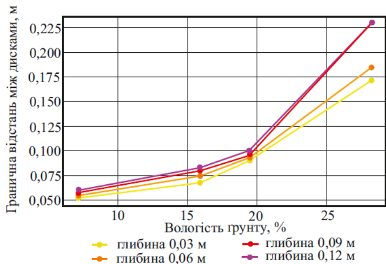
Рис. 1. Залежність граничної відстані між дисками від вологості ґрунту за різної глибини ходу
