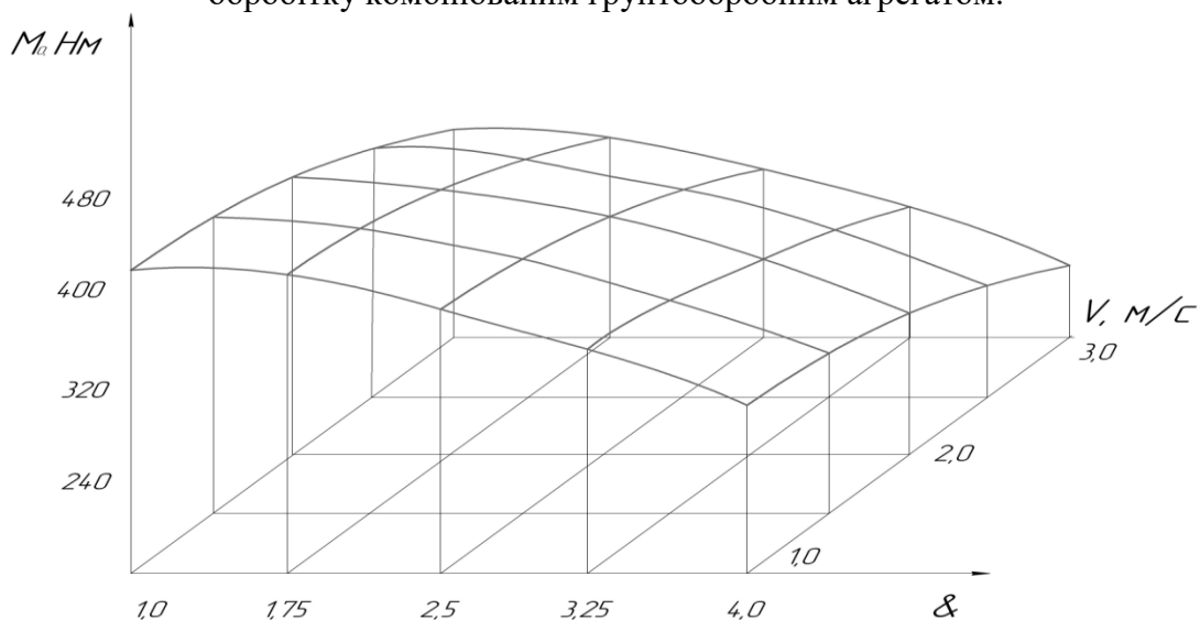
Рис. 3. Зміна моменту опору M_o зубового розпушувача в залежності від поступальної швидкості V і показника кінематичного режиму роботи X зубового розпушувача
