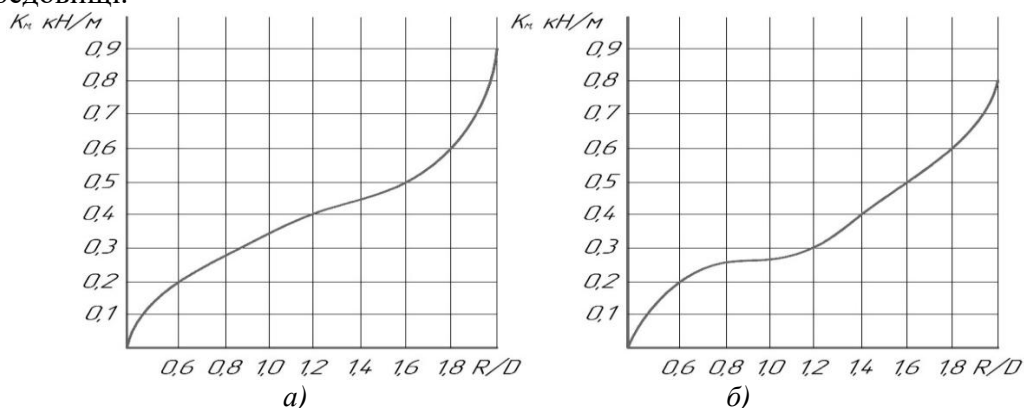
Рис. 2. Залежність питомого тягового опору від співвідношення радіусу сфери до діаметру вирізного диска K_n а - (R/D) , D = 650 мм R=800 мм і кут атаки \alpha = 20^\circ ; б - (R/D) , D = 500 мм R=630 мм і кут атаки \alpha = 20^\circ .
