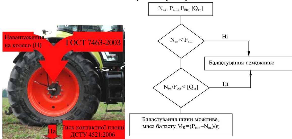
Рис. 4. Обмеження експлуатаційного навантаження на рушій Умова екофільності шини: [5]
