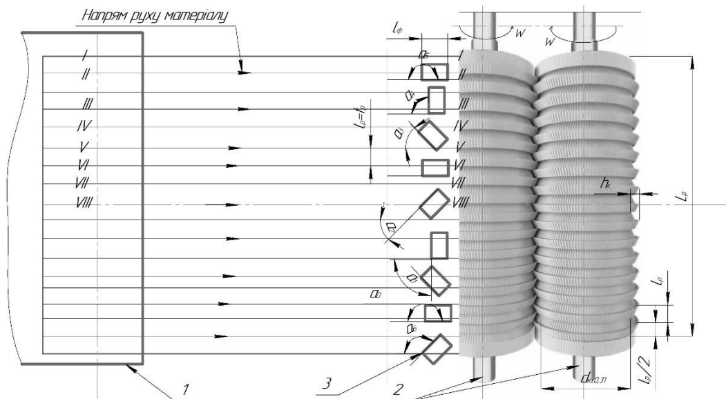
Рис. 2. Розрахунково-технологічна схема подрібнення частіток маси вальцевим подрібнювальним апаратом
