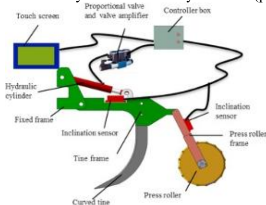
Рис. 2. Електрогідравлічна система керування глибокорихлилем із гнучкими лапами [2]
