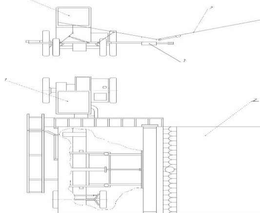
Рис. 1. Схема вібраційної плодозбиральної машини 1 - самохідне шасі ; 2 - уловлювач;
