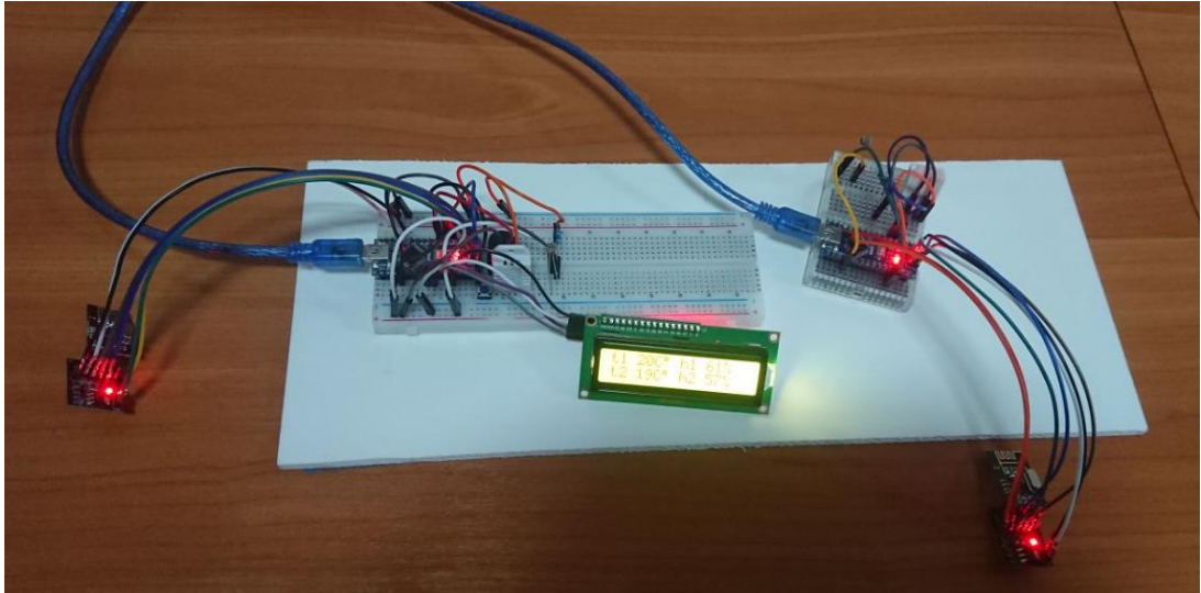
Безпроводна система моніторингу параметрів мікроклімату у теплиці на базі комплексу технічних засобів Arduino
