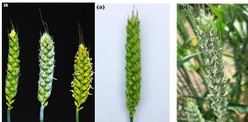
Рис. 1. VAEX-метод
