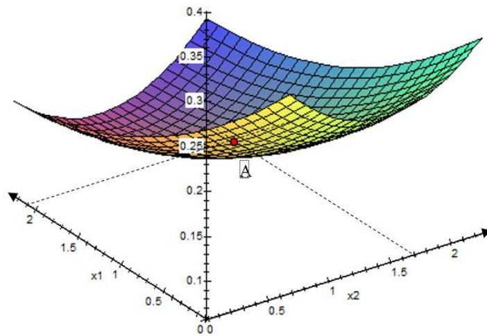
Рис. 4. Поверхня відгуку залежності рівня середніх щодобових втрат плодів вишні у від концентрацій молочної кислоти x_1 та оцтової кислоти x_2
